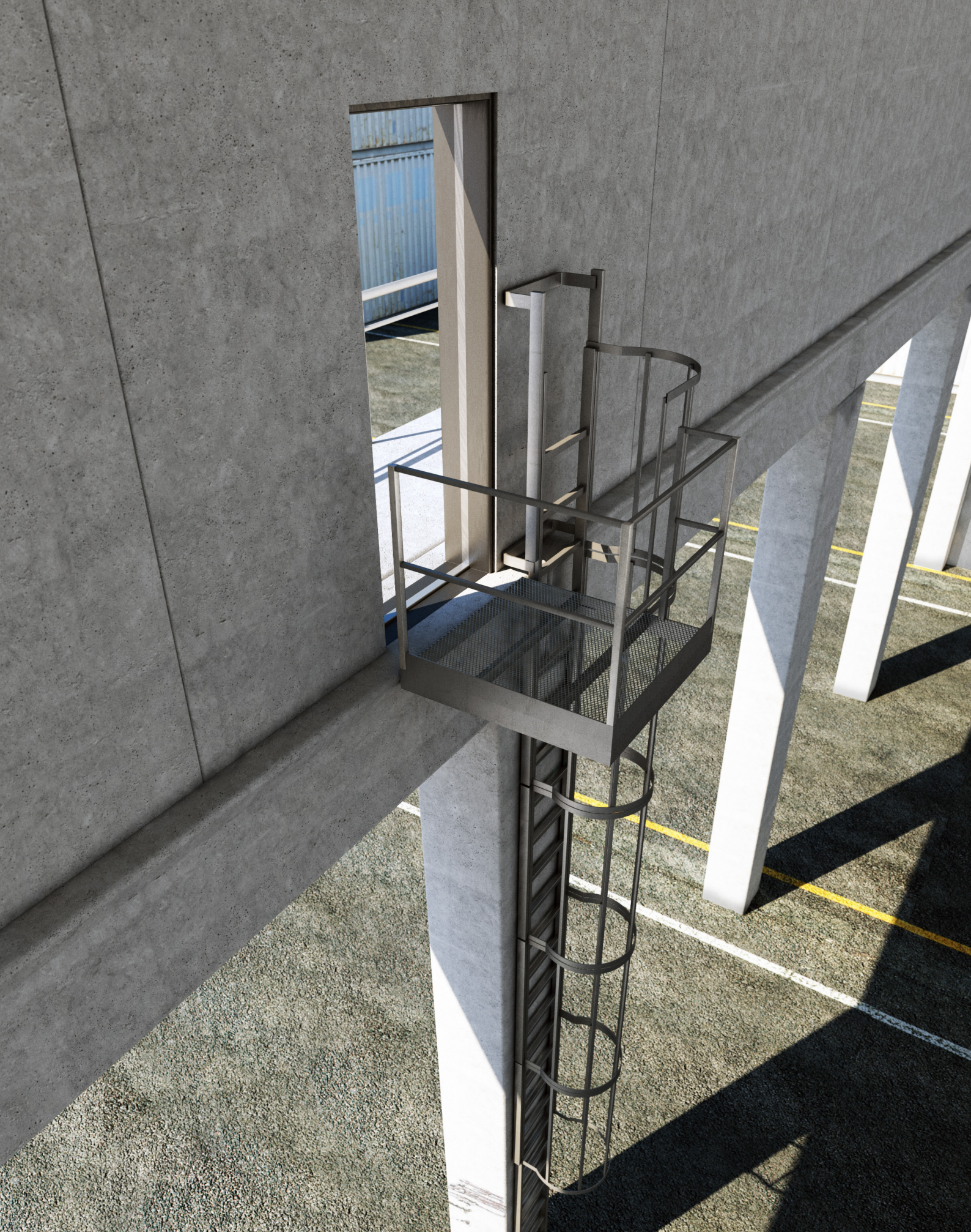
Scala a gabbia con pianerottolo di sbarco laterale
