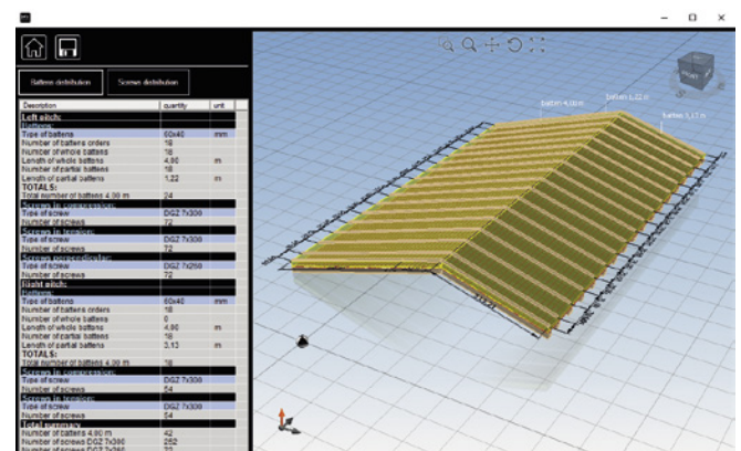
Aufmaß Dachlatten.
