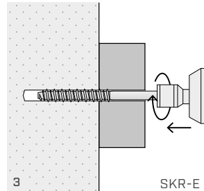
Aseta kiinnitettävä kohde paikalleen ja asenna ruuvi iskuruuvinvääntimellä
