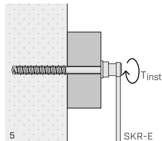
Tarkista kiristysmomentti T_{inst}
