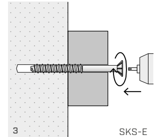
Aseta kiinnitettävä kohde paikalleen ja asenna ruuvi iskuruuvinvääntimellä
