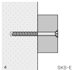
Varmista, että ruuvien kanta on täysin kosketuksessa kiinnitettävään kohteeseen
