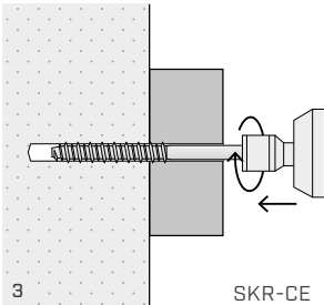
Colocar el objeto a fijar e introducir el tornillo con el atornillador de impulsos
