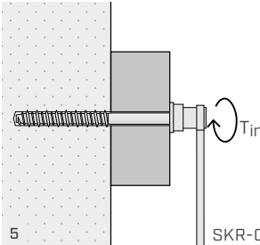
Verificar el par de apriete T_{inst}
