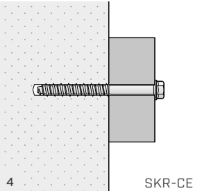
Asegurarse de que la cabeza del tornillo esté bien en contacto con el objeto a fijar
