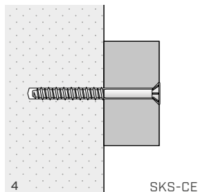
SKS-CE
