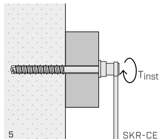
SKR-CE
