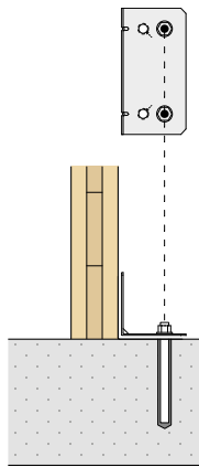
备选安装
