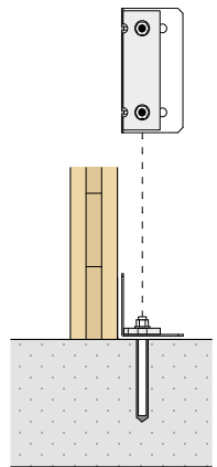
带垫片的安装
