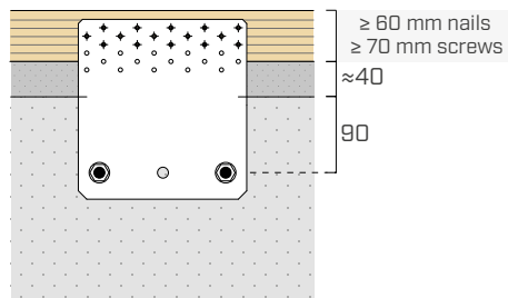
ČIASTOČNÁ 15 UPEVNENÍ - C/GL
