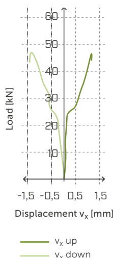
Schémy sily-presunu pri vzorke TCP300 s čiastočným upevnením (14 ks kľincov LBA Ø4 x 60 mm).
