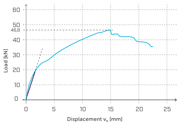
Schémy sily-presunu pri vzorke TCP300 s čiastočným upevnením (14 ks kľincov LBA Ø4 x 60 mm).
