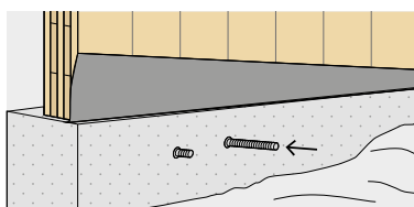
Vstříknutí chemické kotvy a umístění tyčí se závit
