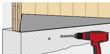
Odstranění desky TITAN TCP a vyvrtání betonu
