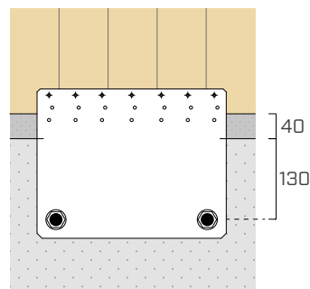
ČÁSTEČNÉ - 7 UPEVNĚVACÍCH PRVKŮ - CLT
