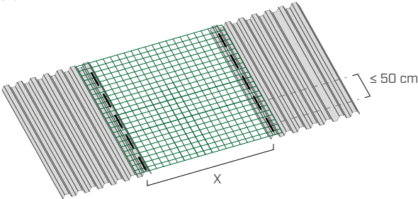
平行梯形/波纹板 安装方案 D
