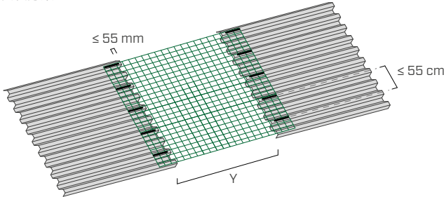
垂直梯形/波纹板 安装方案 E
