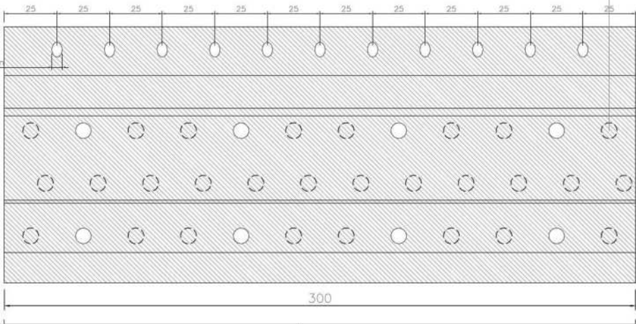
BASIC MODULE
