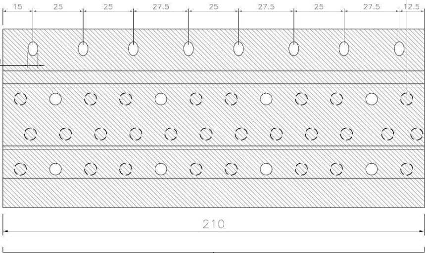
BASIC MODULE
