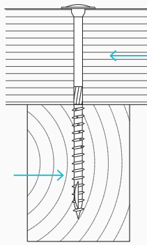
木-木
