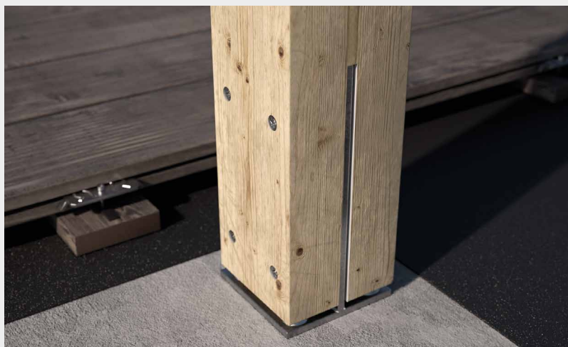
^ Pričvršćenje nosača stupa Rothoblaas s unutarnjim perom F70.
