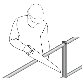
12 - Adaptar la última sección cortando la parte sobrante.
