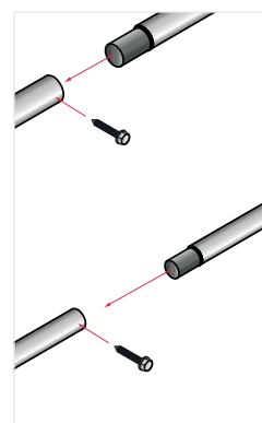
10 - Insérer les lisses et les sous-lisses des sections montées avec des vis 4,8 x 16.
