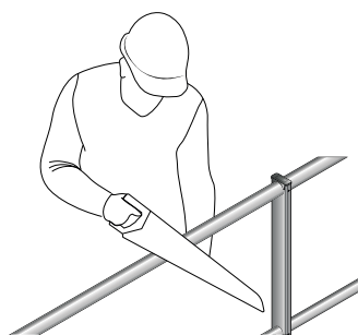
12 - Adattare l'ultima sezione tagliando la parte in eccedenza.
