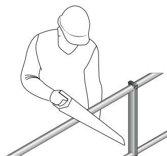
12 - Den letzten Abschnitt anpassen, indem das überstehende Teil abgeschnitten wird.
