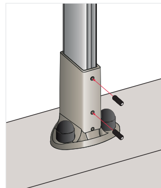
6 - Apretar los tornillos prisioneros.
