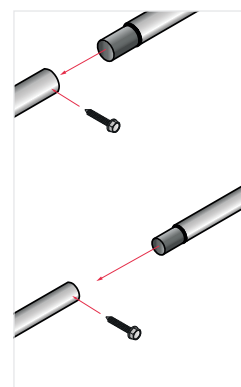
10 - Inserire i corrimani e i correnti intermedi delle sezioni montate con viti 4,8 x 16.
