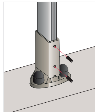
6 - Serrer les vis sans tête.
