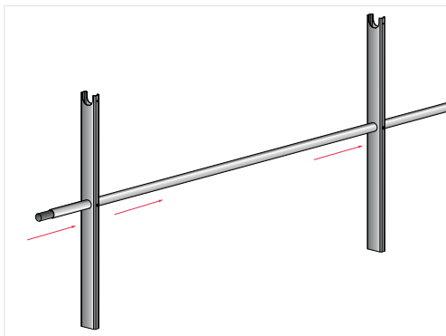
4 - Insérer une sous-lisse dans 2 montants.
