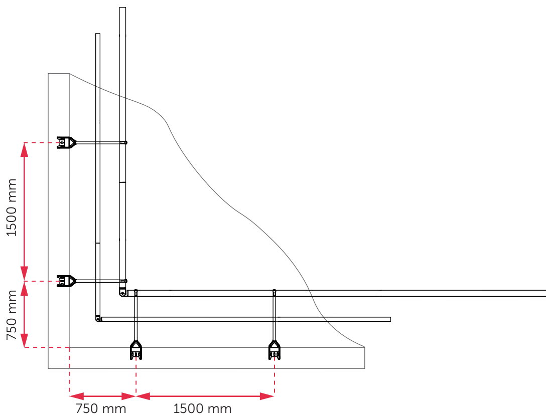
MONTANTS INCLINÉS
