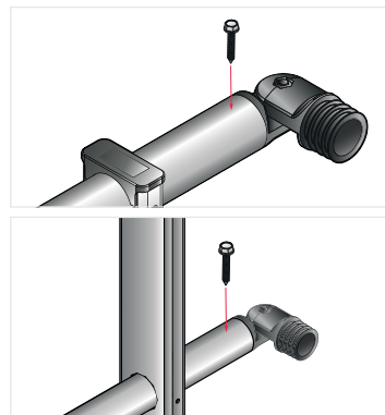
12 - Fixer les angles avec des vis autoforeuses 4,8 x 25.
