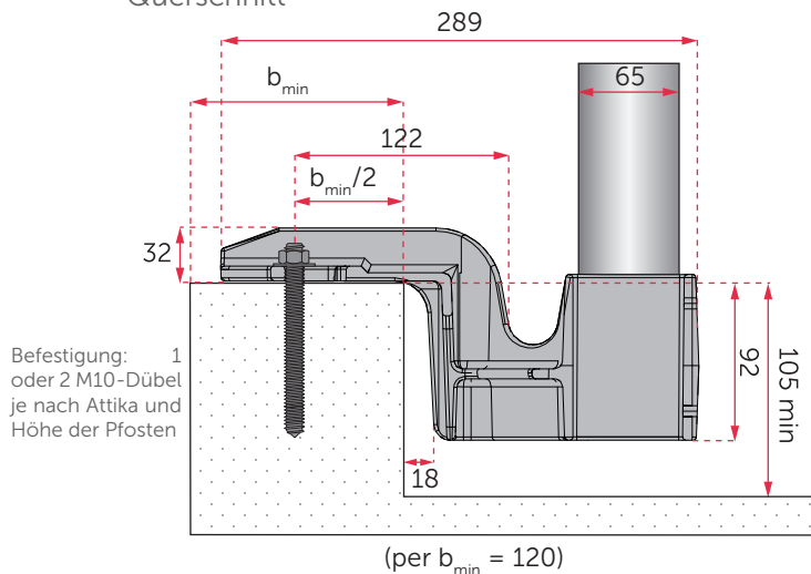
Querschnitt
