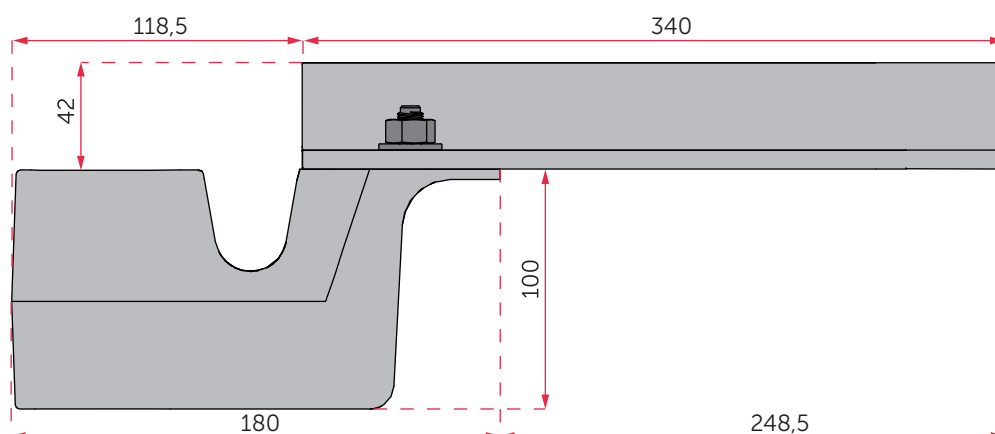
Vue latérale
