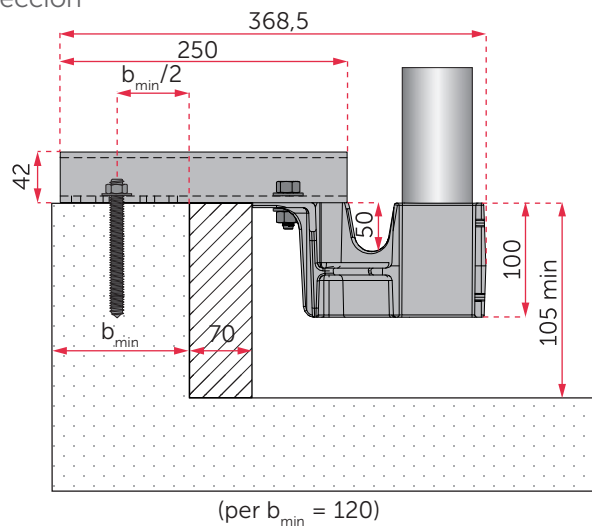
Sección
