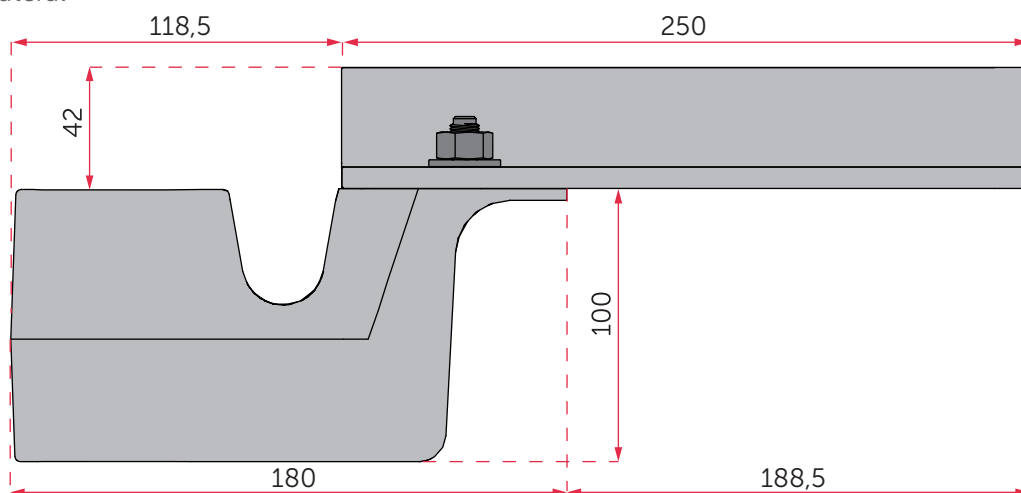
Vista lateral
