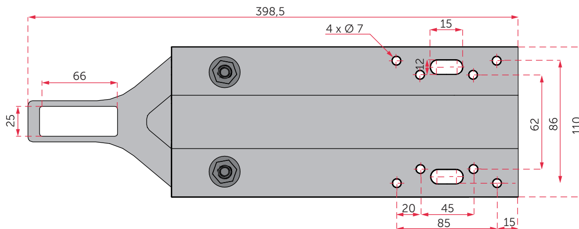
Draufsicht
