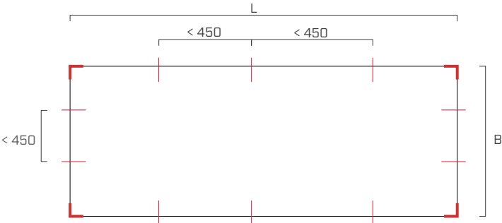
Distanze massime per il posizionamento delle staffe di fissaggio
