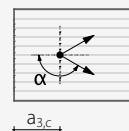
extremidade sem carga 90^\circ < \alpha < 270^\circ
