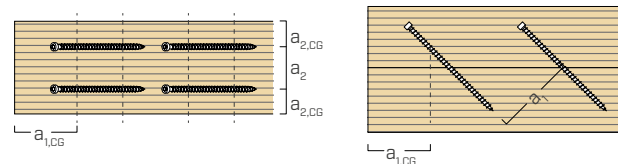
půdorys
