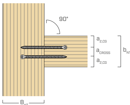
půdorys - 1 PÁR
