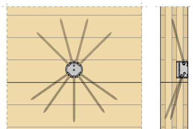
δάπεδο-δάπεδο | τοίχος-τοίχος
