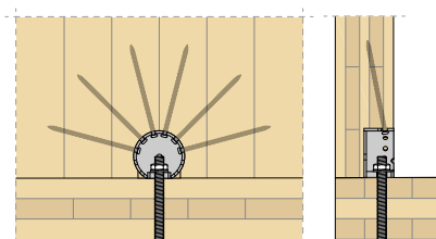
ξύλο-ξύλο
