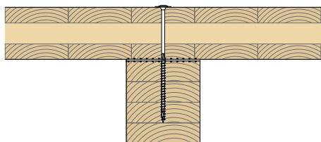
Befestigung mit Schrauben
