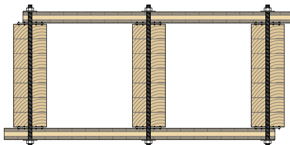
Befestigung mit Gewindestangen oder Bolzen
