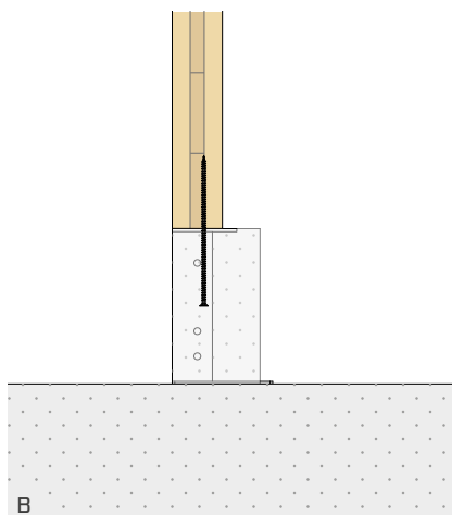
B TC FUSION AVEC INSERTION PAR LE BAS
