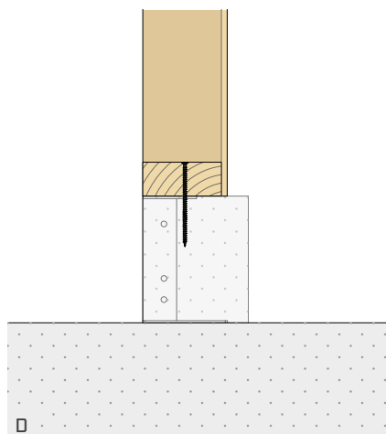
D TC FUSION AVEC INSERTION PAR LE HAUT
