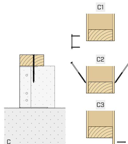
C TC FUSION AVEC POUTRE DE BASE
