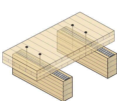
(A) SECÇÕES COMPOSTAS
