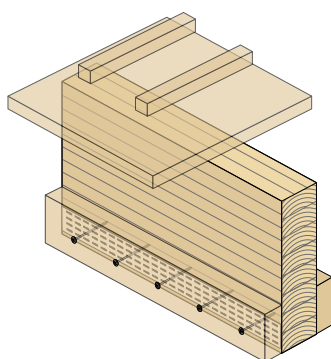
(B) REFORÇO ESTRUTURAL
