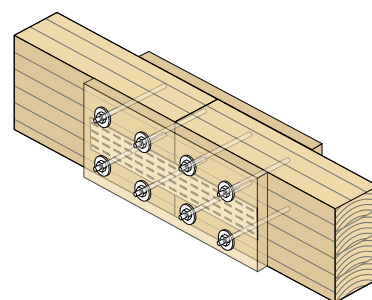
(C) ENRIJECEMENTOS LOCAIS DAS JUNTAS
