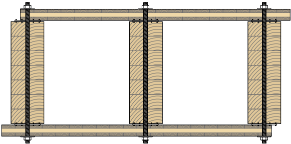
fixação com barras roscadas ou parafusos
