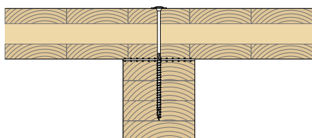
rögzítés csavarral
