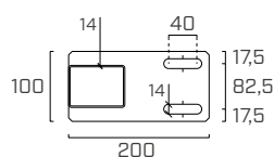
spodnja plošča
