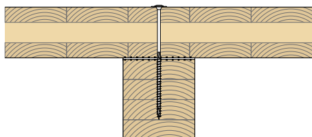
pričvršćenje vijcima
