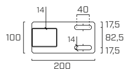
dolní deska
