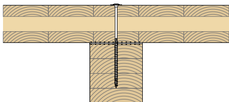
upevnění vruty
