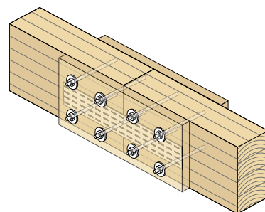
(С) ЛОКАЛЬНОЕ ПОВЫШЕНИЕ ЖЕСТКОСТИ СОЕДИНЕНИЙ
