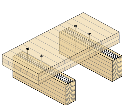
(А) СОСТАВНЫЕ СЕКЦИИ
