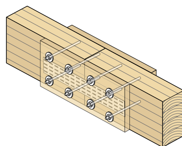
(C) LOKÁLNÍ VYZTUŽENÍ SPOJŮ
