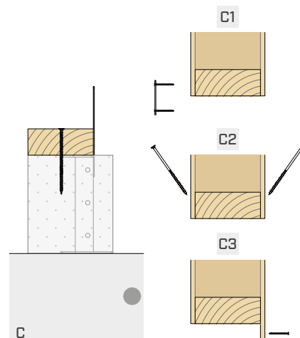
TC FUSION TÁMASZTÓGERENDÁVAL
