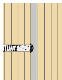
Trucioli che ostruiscono i fori nell'acciaio durante la foratura (distanziatori non installati).
