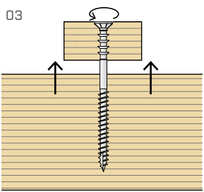
Dévisser en fonction de la distance souhaitée.
