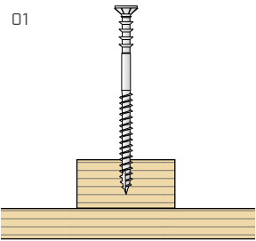
Positionner la vis DRS.
