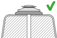
Atornillado correcto
