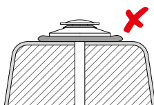
过度拧紧
