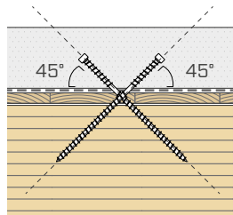
45° - os kereszttezett telepítés hangszigetelő lemezzel vagy anélkül.
