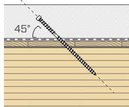
45° - os telepítés hang-szigetelő lemezzel.
