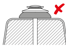
Nedostatočné skrutkovanie
