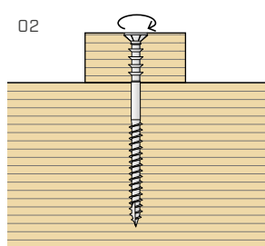
Upevnenie lišty zaskrutkovaním skrutky tak, že hlava je v jednej rovine s dreveným prvkom.
