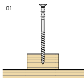
Umiestnenie skrutky DRS.
