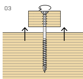
Uvoľnenie skrutky podľa požadovanej vzdialenosti.
