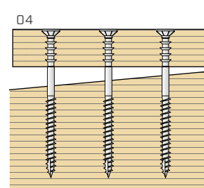
Nastavenie ostatných skrutiek rovnakým spôsobom pre vyrovnanie konštrukcie.
