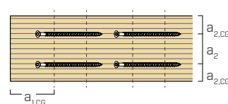
půdorys
