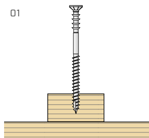
Aseta DRS-ruuvi.
