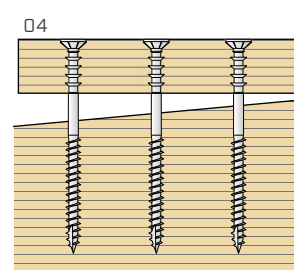
Säädä muut ruuvit samalla tavalla rakenteen tasaamiseksi.
