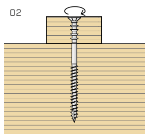
Kiinnitä lista kiristämällä ruuvia niin, että kanta on samassa tasossa puuelementin kanssa.
