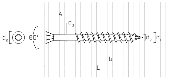
SHSAS Ø3,5
