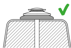
Correcte montage
