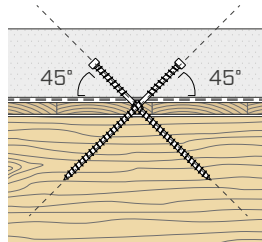
Kruislingse installatie op 45° met of zonder geluidsisolerende laag.
