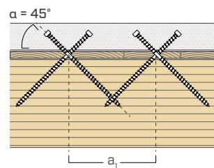
45° kryssende
