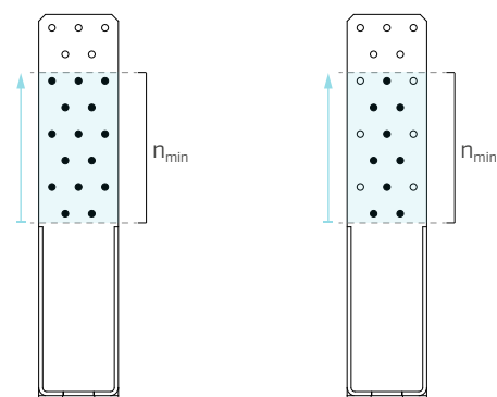
WHT20: fixare parțială în configurația wide pattern și respectiv narrow pattern, cu instalarea numărului minim de conectori n_{min} .
