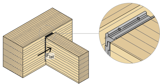
κεκλιμένη βίδα
