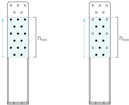
WHT20: μερική στερέωση στη διαμόρφωση wide pattern και narrow pattern αντίστοιχα με εγκατάσταση του ελάχιστου αριθμού συνδέσμων n_{\min} .
