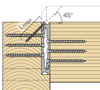
дополнительный шуруп Ø5 мм - L_{max} = 50 мм
