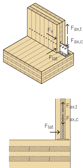
соединение стены CLT с перекрытием CLT
