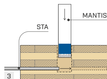
3 Inserire spinotto STA e MANTIS
