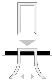
interner Schnitt
