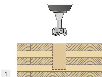
1 Perçer le trou borgne supérieur
